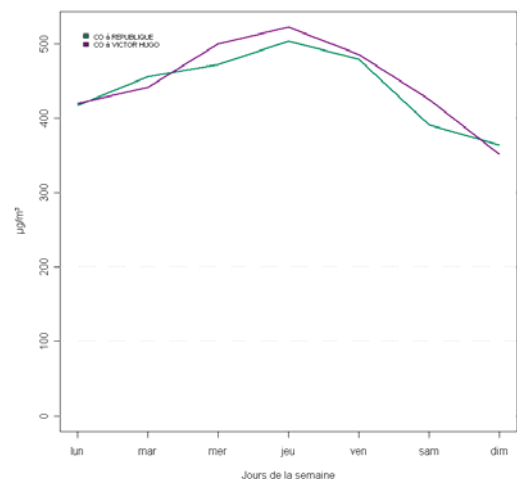
Graphique 21 : évolution hebdomadaire des niveaux de monoxyde de carbone
