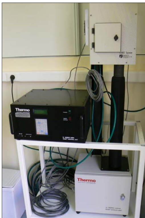
Photo 2 : un analyseur de particules TEOM équipé d'un module additionnel FDMS
