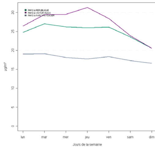
Graphique 20 : évolution hebdomadaire des niveaux de particules PM 10
