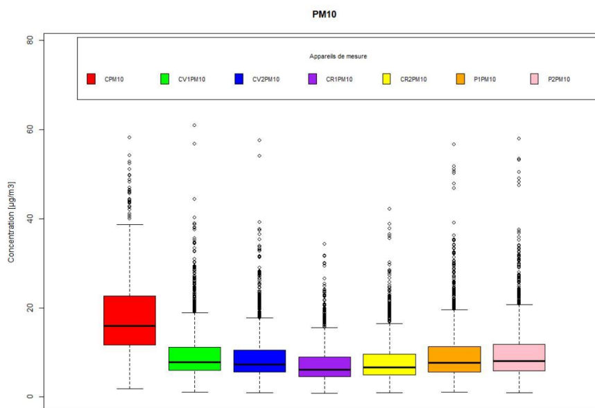
Figure 17 : boxplot des mesures en PM 10 par l'analyseur de référence (en rouge, à gauche) et par les microcapteurs.
