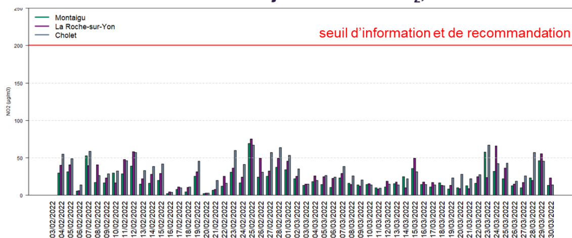
Figure 5 : maxima horaires journaliers des concentrations en NO 2 au cours de la phase estivale (en haut) puis hivernale (en bas)
