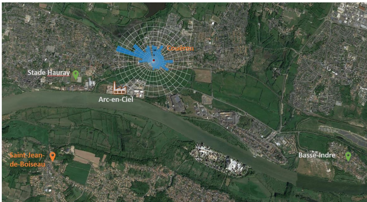
Figure 17 : rose de pollution moyenne
