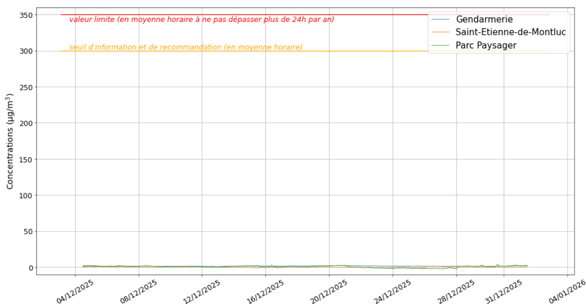
Figure 25 : évolution des concentrations maximums horaires journalières en SO 2 sur les 3 sites de mesure, dont 2 non influencés par l'UVE
