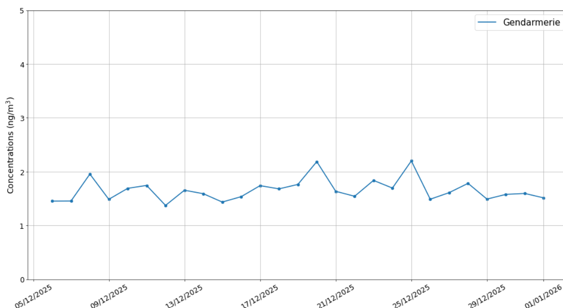
Figure 30 : évolution de la concentration du maximum horaire journalier en mercure gazeux au cours de la campagne hivernale de 2025, sur le site de la Gendarmerie à Couëron
