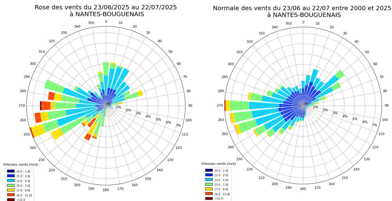
Figure 3 : rose des vents au cours de la campagne estivale (à gauche) et rose des vents normale (à droite), du 23 juin au 22 juillet 2025. Source : Météo-France
