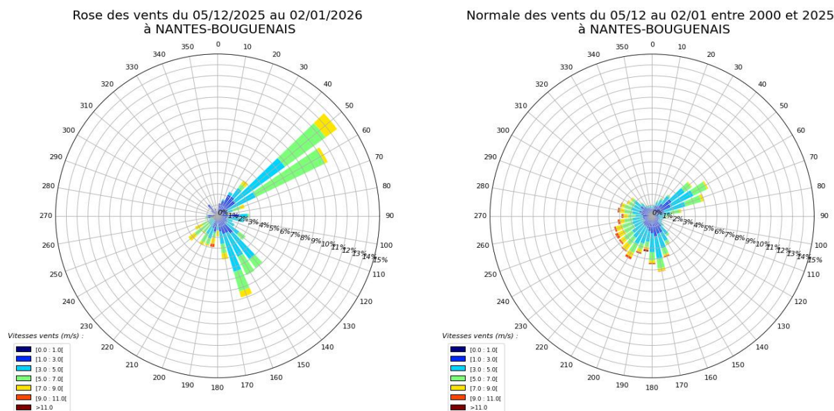
Figure 5 : rose des vents au cours de la campagne hivernale (à gauche) et rose des vents normale (à droite), du 5 décembre 2025 au 2 janvier 2026. Source : Météo-France
